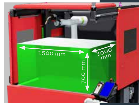
Bauteildimensionen ohne Dreheinheit
